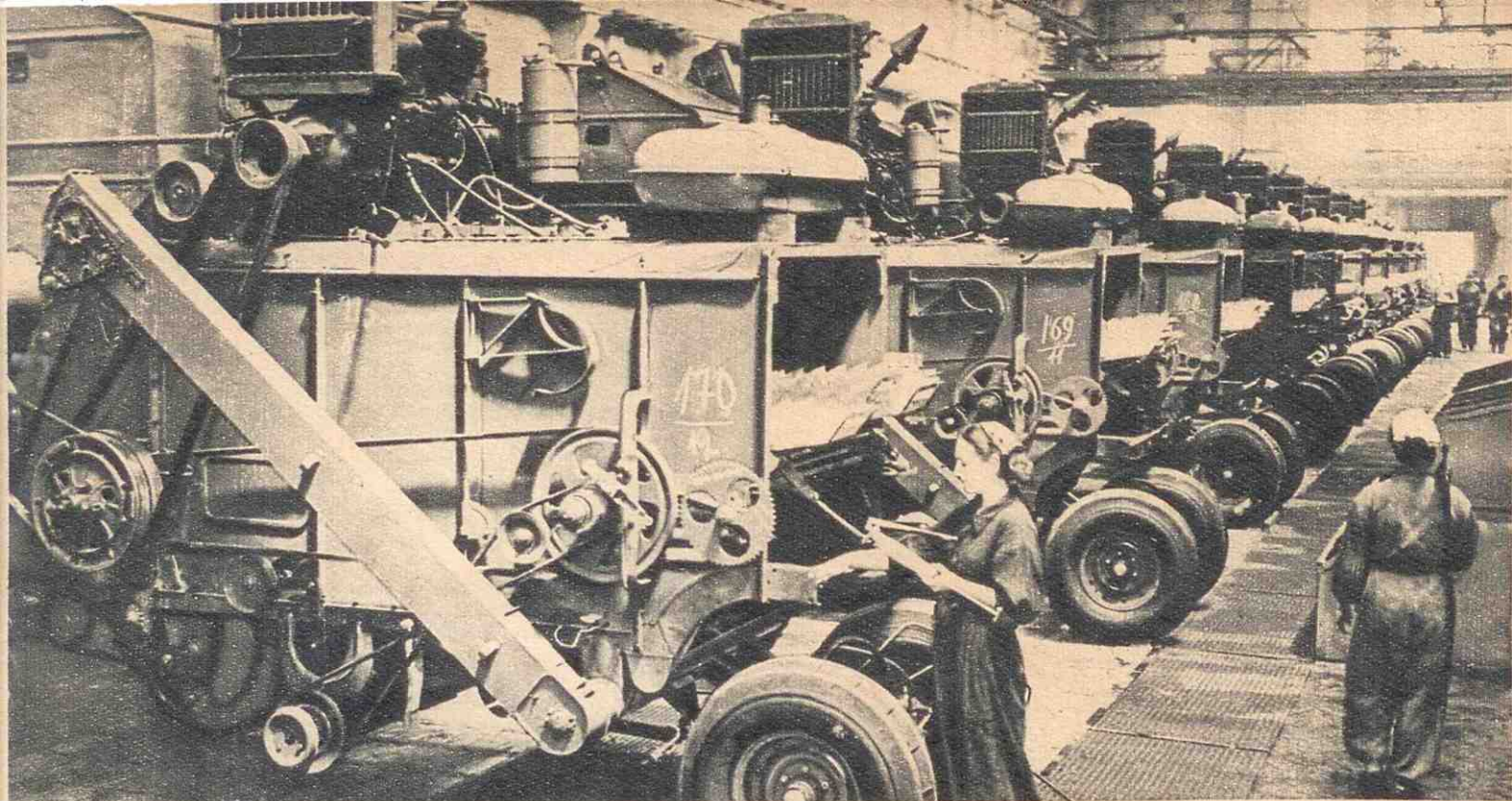
Сборка комбайнов.
